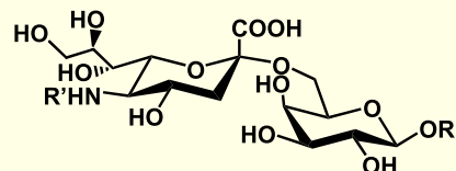
Neu5Aα(2-3/6)Gal Neu5Gα(2-3/6)Gal
