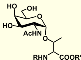
GalNAc-Ser / Thr
